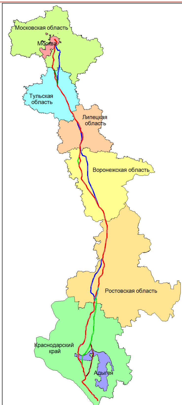
Рисунок 2.1. Схема рассматриваемых в ОВОС вариантов ВСМ Центр-Юг.
