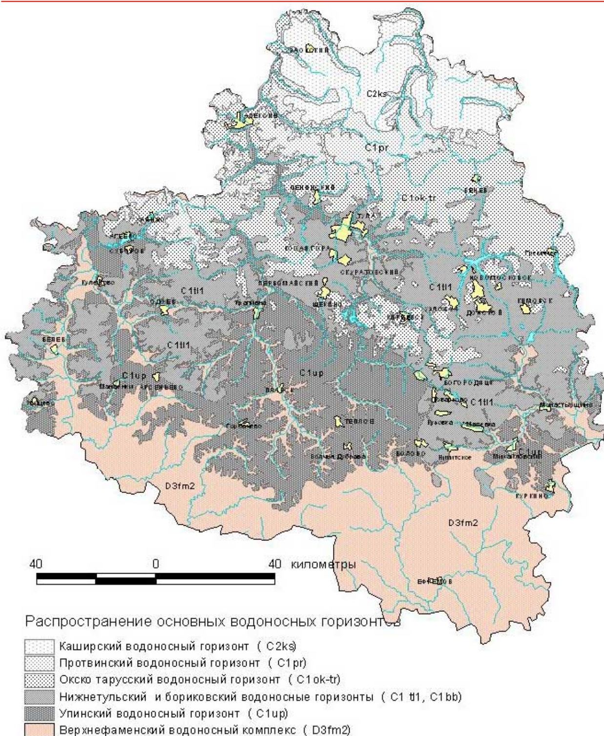
Рисунок 5.2.1. Схематическая карта распространения основных эксплуатационных водоносных горизонтов в пределах Тульской области
